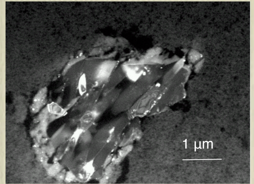
FeS crystal
