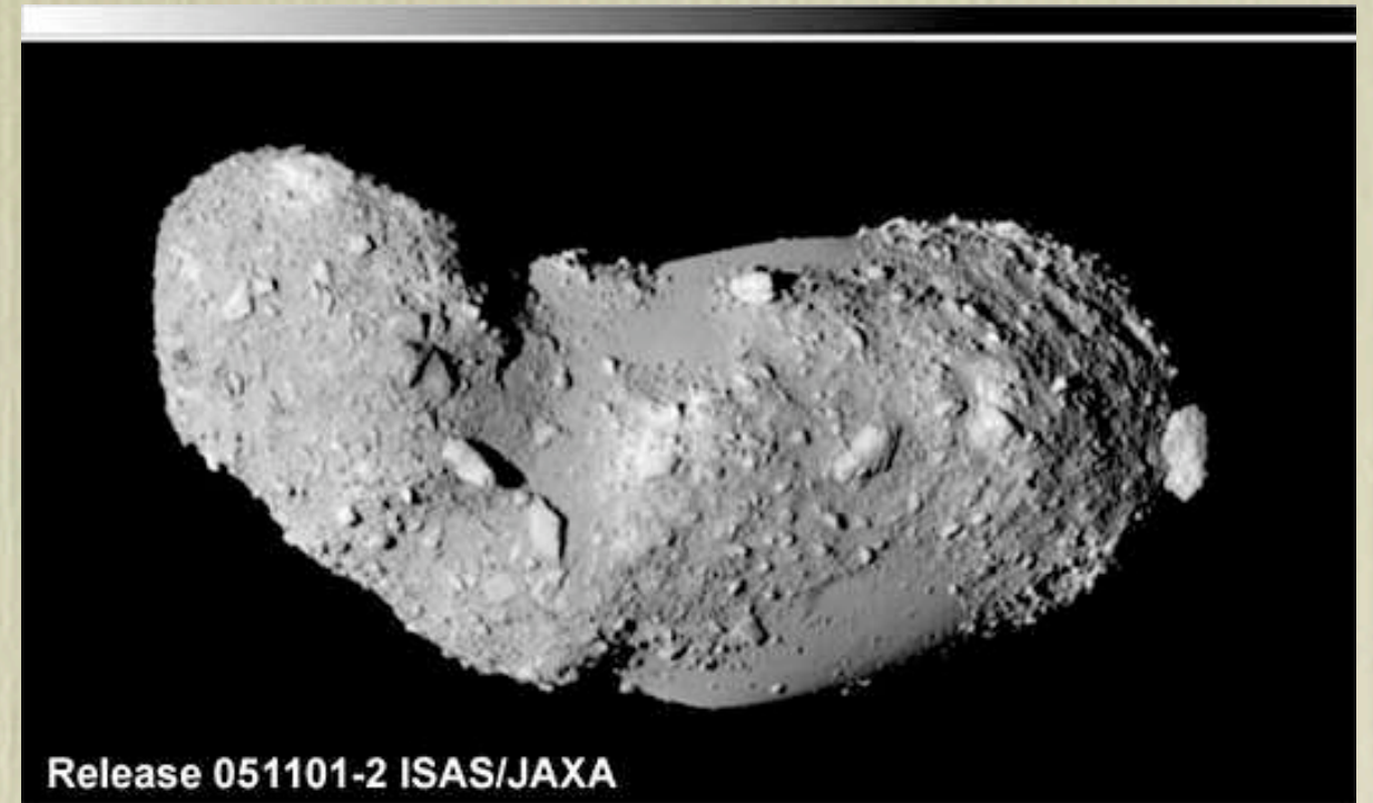
Itokawa
